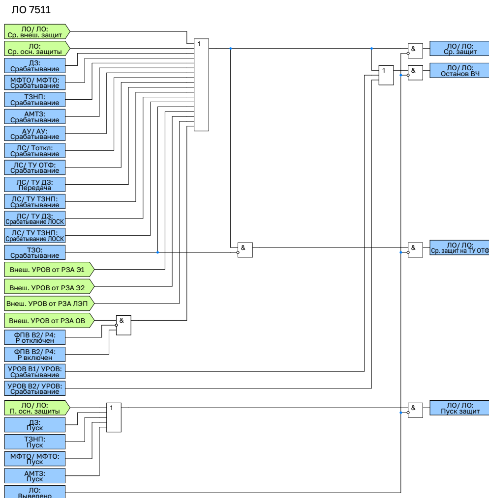
Рисунок 2.56 – Функциональная схема общей логики отключения
