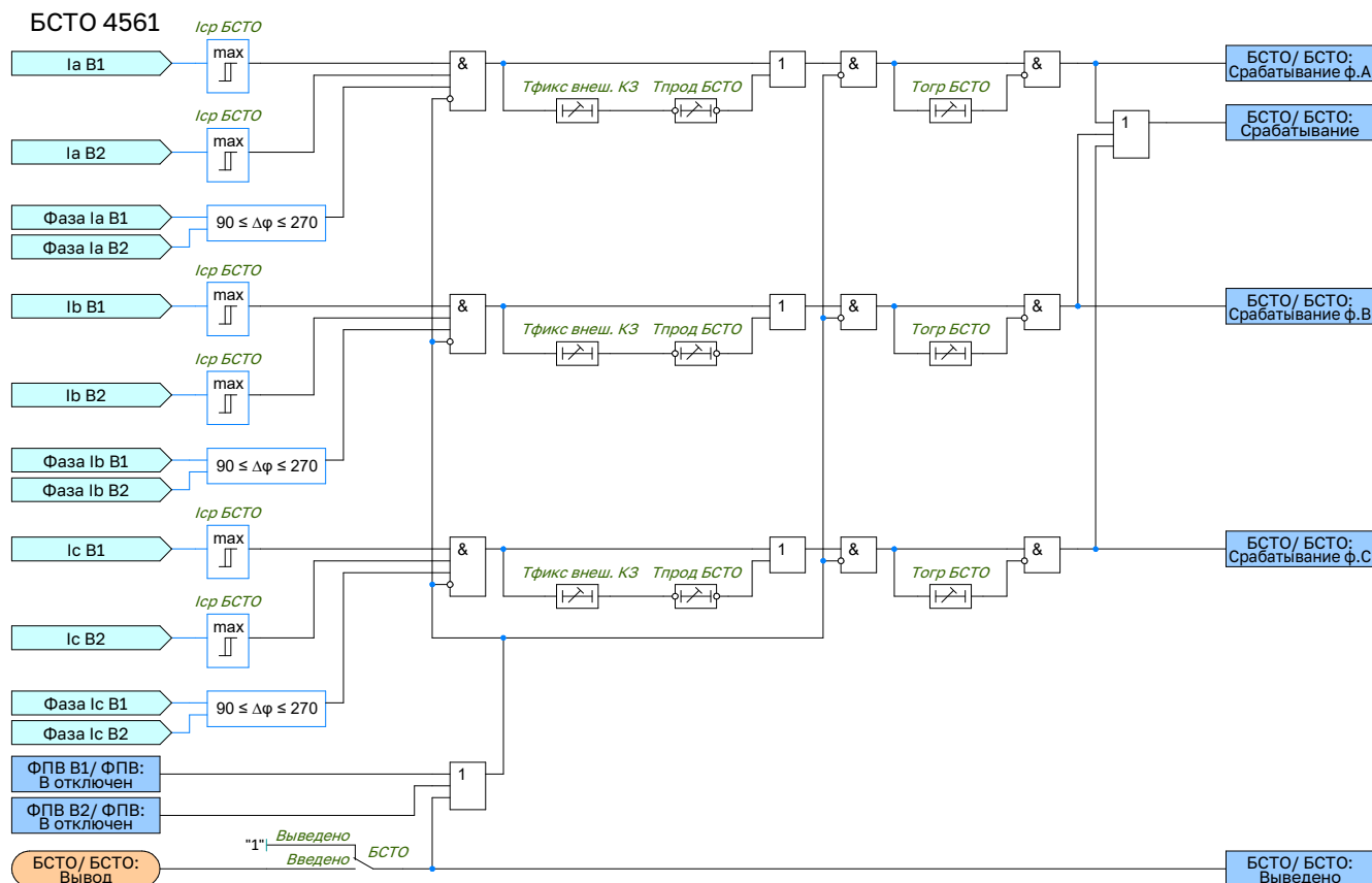
Рисунок 2.33 – Функциональная схема БСТО
