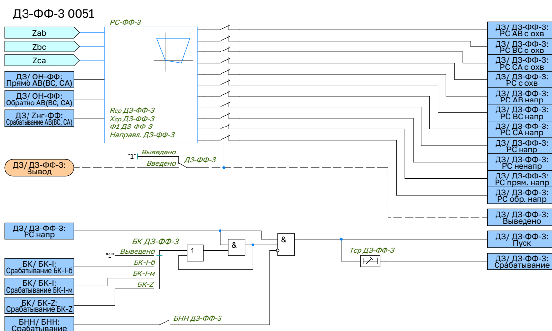
Рисунок 2.12 – Функциональная схема логики ДЗ-ФФ-3
