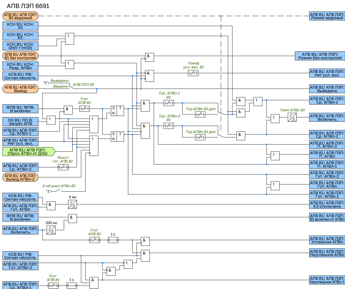
Рисунок 2.46 – Функциональная схема логики АПВ В1 ЛЭП
