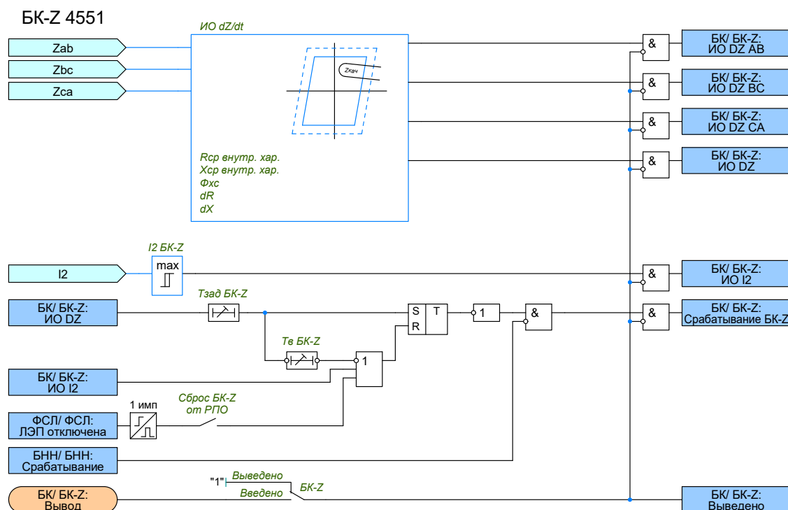
Рисунок 2.19 – Функциональная схема БК-Z
