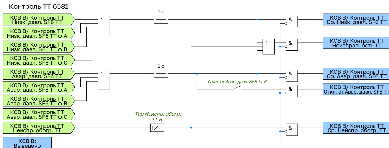
Рисунок 2.52 – Функциональная схема логики контроля ТТ выключателя
