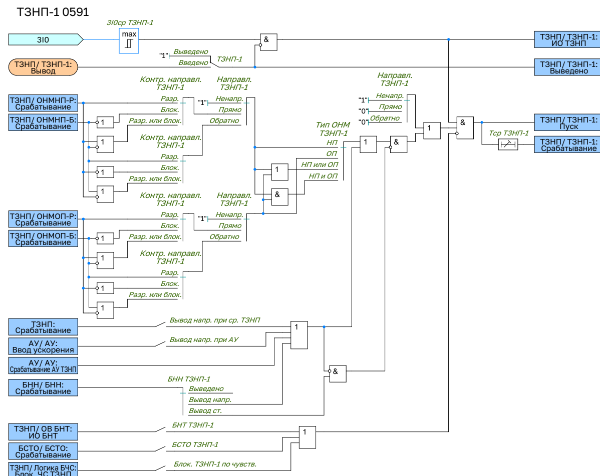
Рисунок 2.21 – Функциональная схема ступени ТЗНП-1
