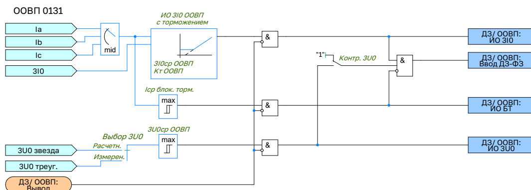
Рисунок 2.9 – Функциональная схема логики ООВП
