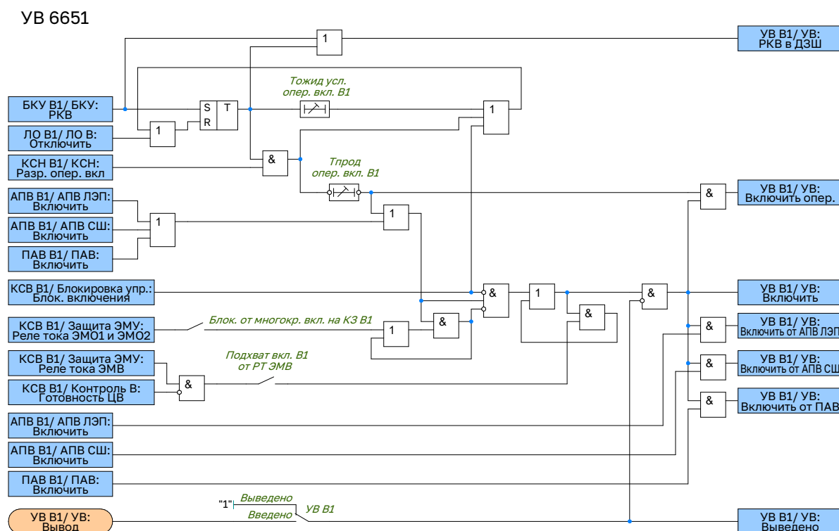
Рисунок 2.59 – Функциональная схема управления выключателем В1
