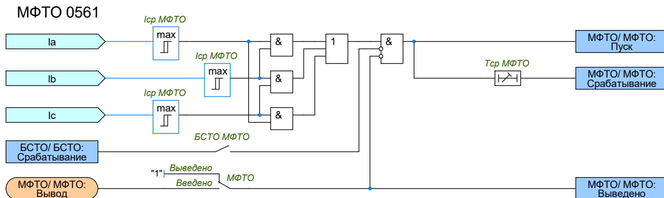
Рисунок 2.29 – Функциональная схема МФТО
