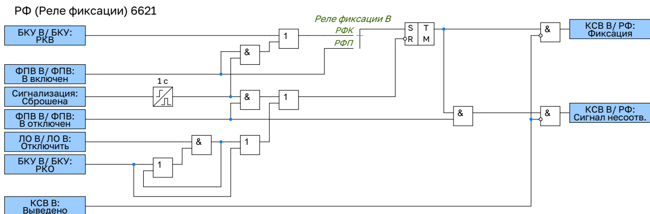
Рисунок 2.55 – Функциональная схема логики реле фиксации выключателя
