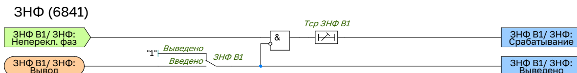
Рисунок 2.34 – Функциональная схема ЗНФ
