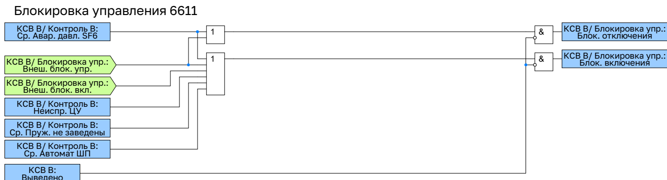
Рисунок 2.54 – Функциональная схема логики блокировки управления выключателя
