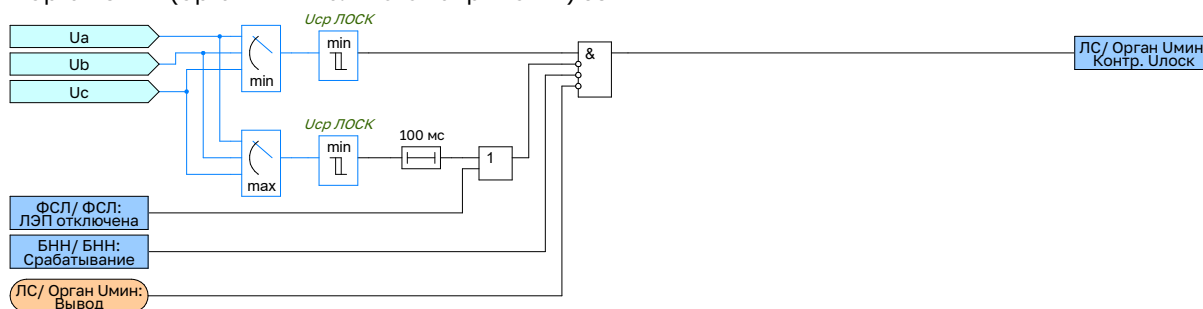
Рисунок 2.42 – Функциональная схема логики контроля минимального напряжения ЛОСК
