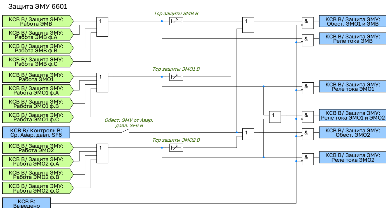
Рисунок 2.53 – Функциональная схема логики защиты ЭМУ выключателя
