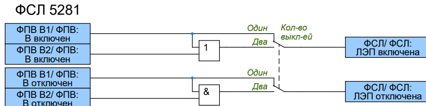
Рисунок 2.65 – Функциональная схема логики ФСЛ
