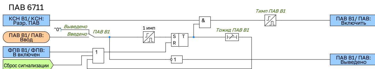
Рисунок 2.50 – Функциональная схема логики ПАВ В1
