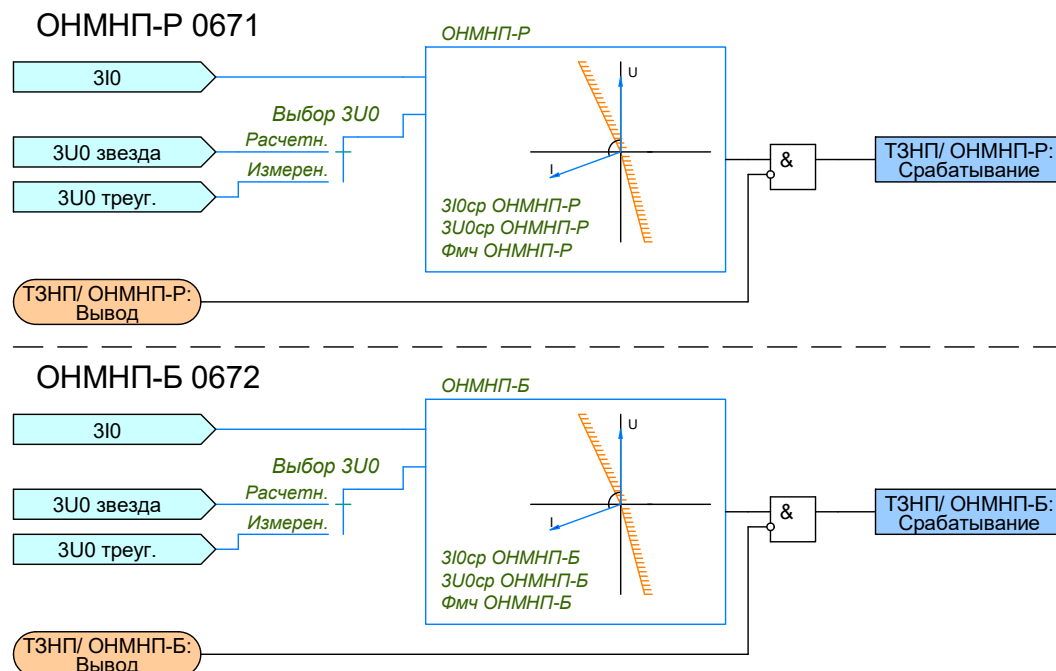
Рисунок 2.24 – Функциональная схема логики ОНМНП
