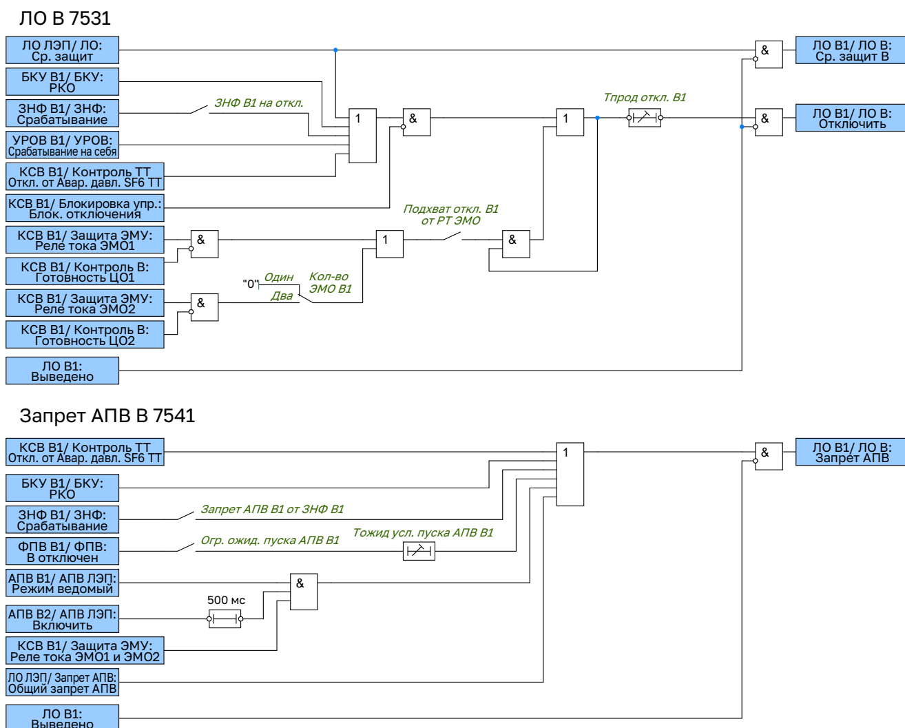
Рисунок 2.58 – Функциональная схема логики отключения В1 и запрета АПВ В1
