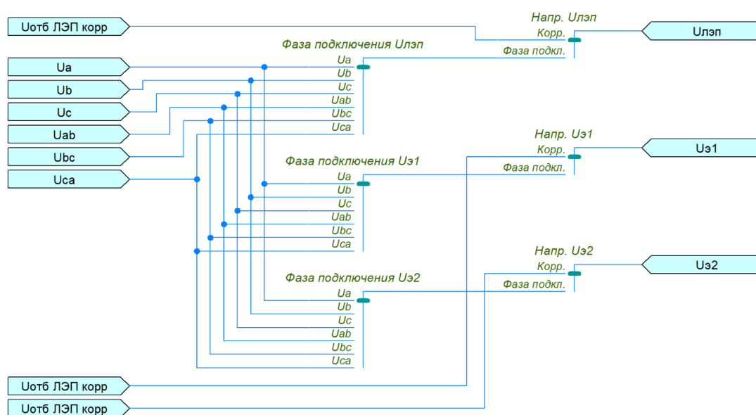
Рисунок 2.67 – Функциональная схема настройки аналоговых значений U_{ЛЭП} , U_{Э1} , U_{Э2}
