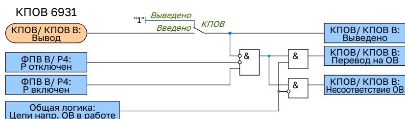
Рисунок 2.66 – Функциональная схема логики контроля перевода на ОВ
