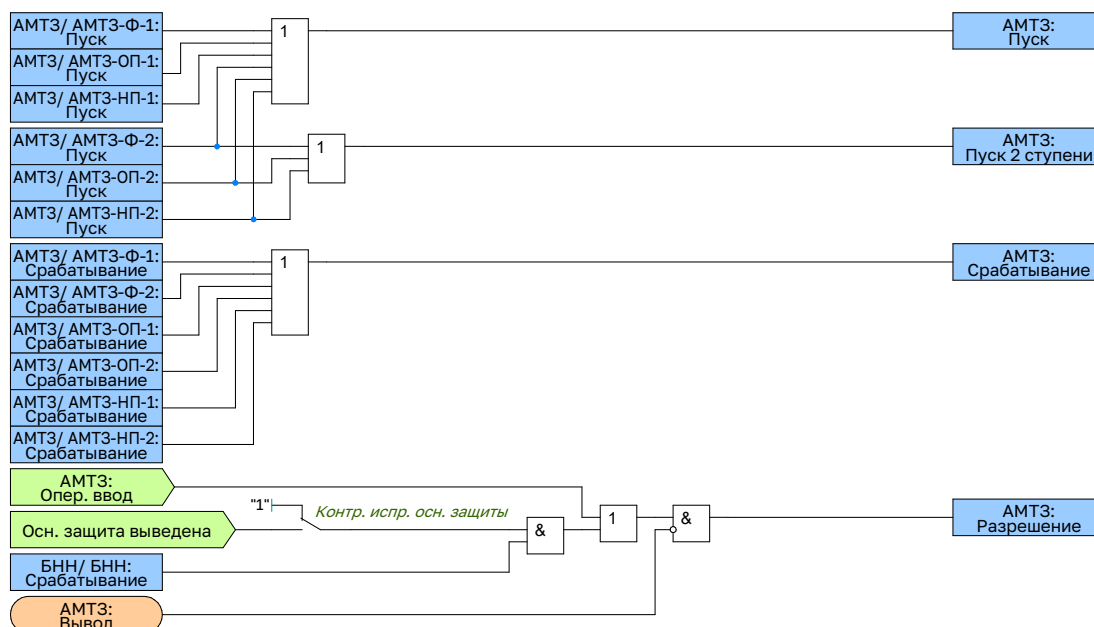
Рисунок 2.31 – Функциональная схема общей логики АМТЗ
