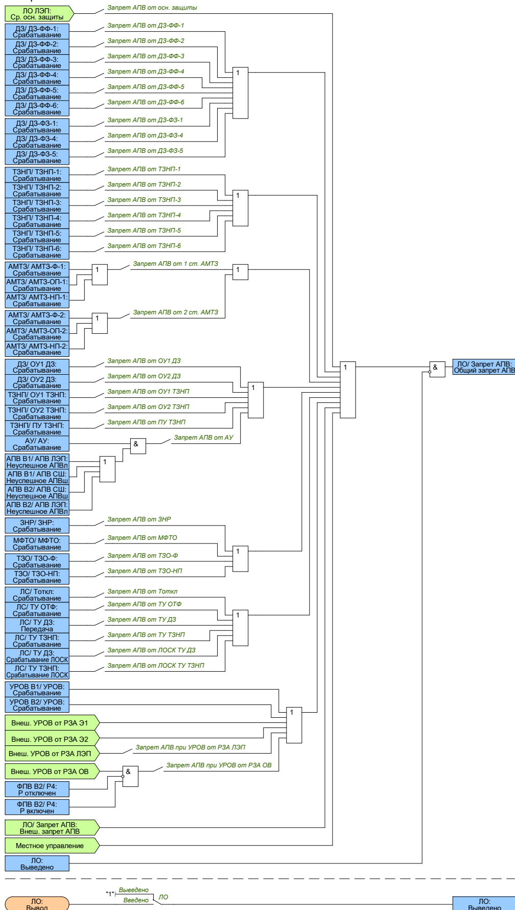
Рисунок 2.49 – Функциональная схема общего запрета АПВ
