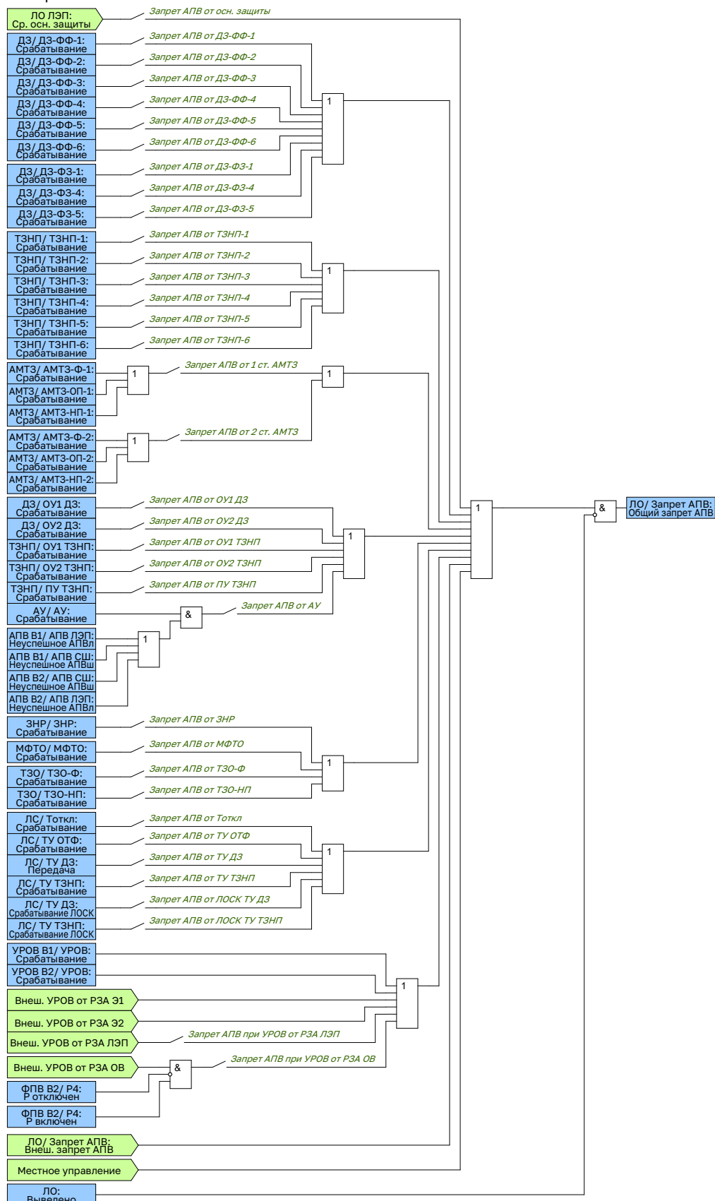
Рисунок 2.57 – Функциональная схема общей логики запрета АПВ
