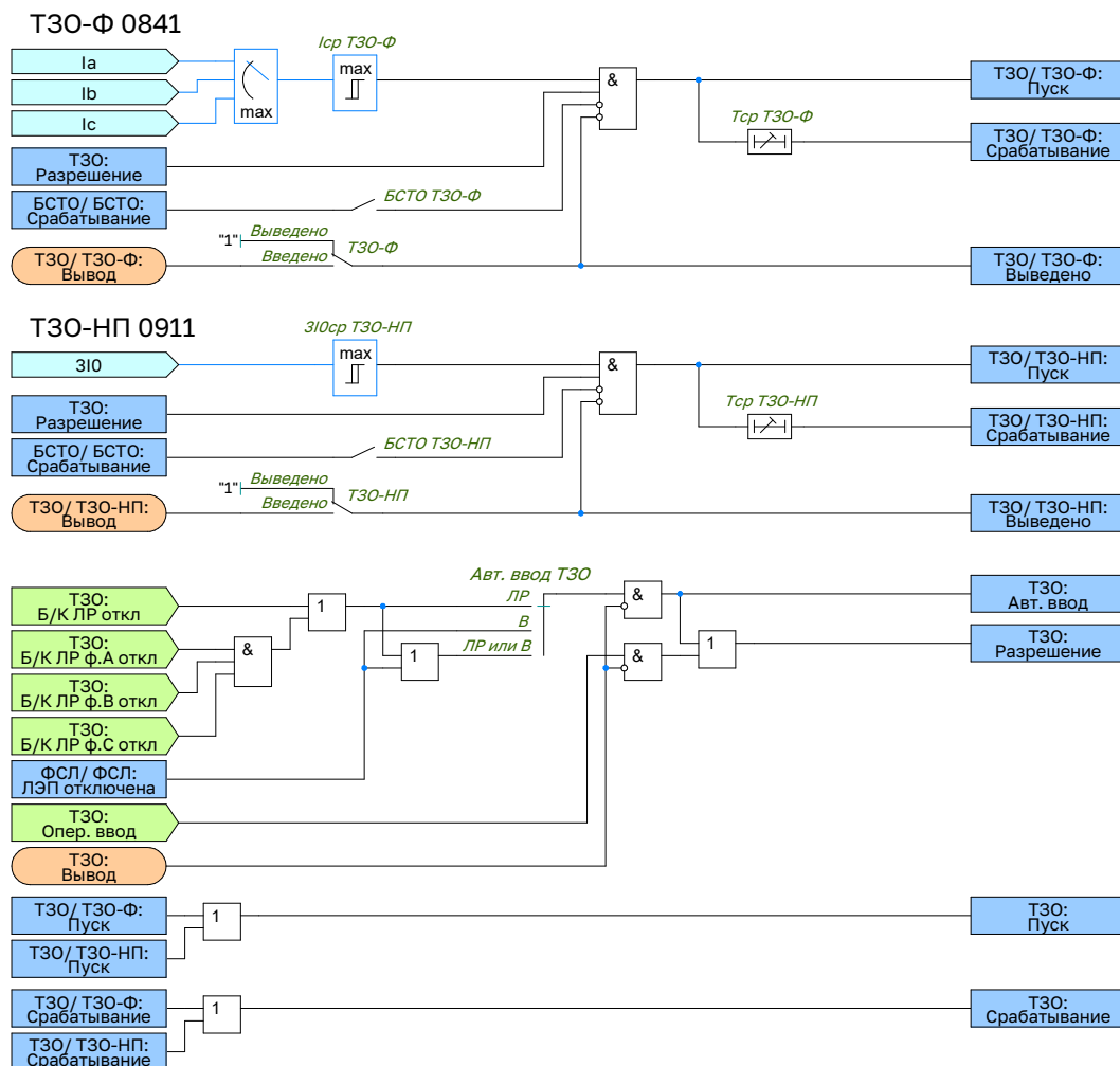
Рисунок 2.32 – Функциональная схема ТЗО
